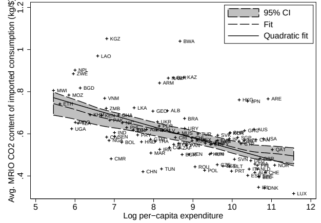
(d) Total \text{CO}_2 content of imports
